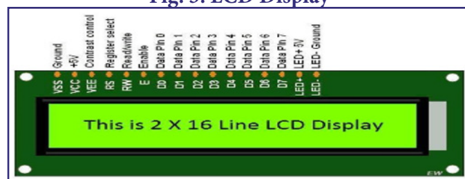
Fig. 3: LCD Display
